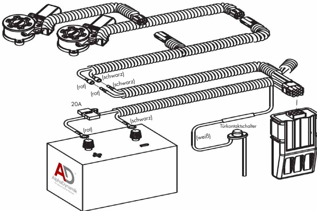
Abbildung 4: Elektrokomponenten bis Mai 2021
