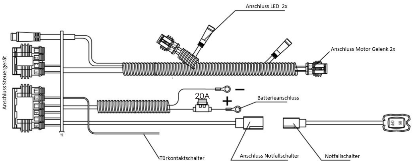
Abbildung 4a: Elektrokomponenten ab Mai 2021
