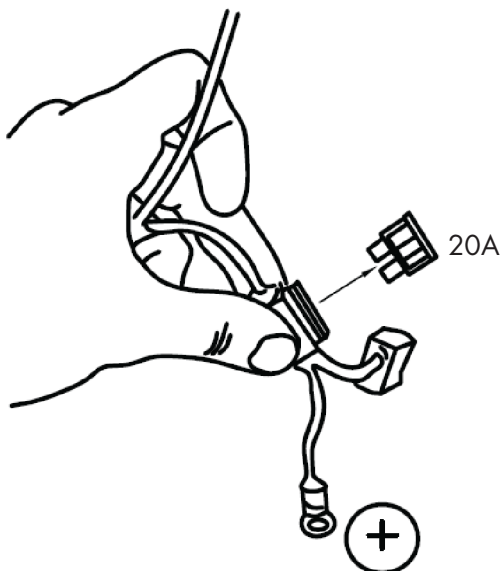
Abbildung 6: Sicherung entfernen!
