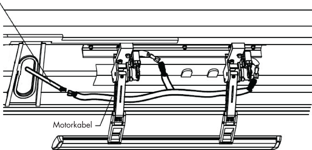
Abbildung 7: Steckverbindung Motorkabel Innen-Außen
