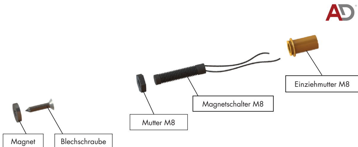
Abbildung 8: Aufbau Türkontakt Universell
